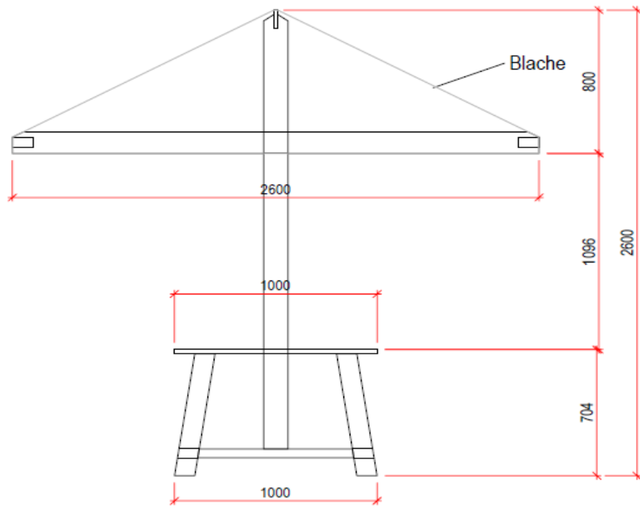
Seitenschnitt
